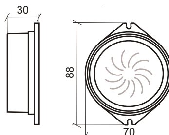
Рис.2 Габаритные и установочные размеры
