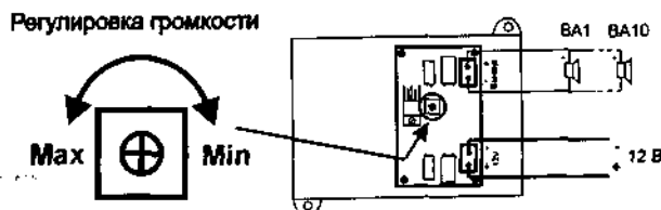
Рис.2 Схема подключения ПКИ-РО.
