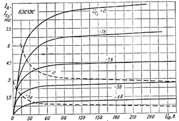
Рис. 211. Усредненные характеристики зависимости тока анода от напряжения на аноде при напряжении на первой сетке — 3 в и напряжении на третьей сетке 0.
