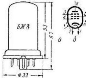
Лампа 6Ж8:
