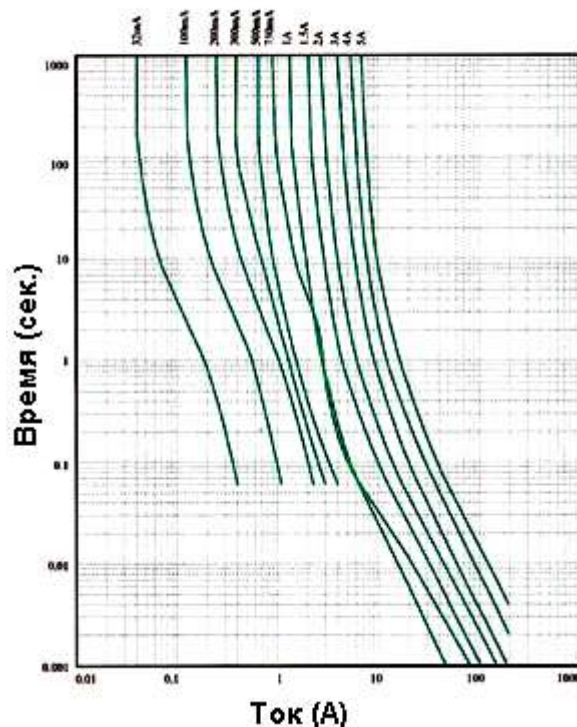
Токовременная зависимость
