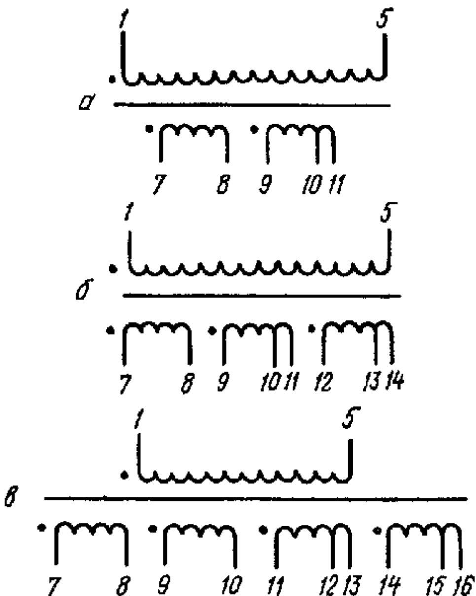
Рисунок 2. Электрические принципиальные схемы накаливающих трансформаторов ТН на 50 Гц, 220 В на броневых сердечниках ШЛ и ШЛМ: а - ТН1...ТН11. б - ТН12...ТН29; в - ТН30...ТН61
