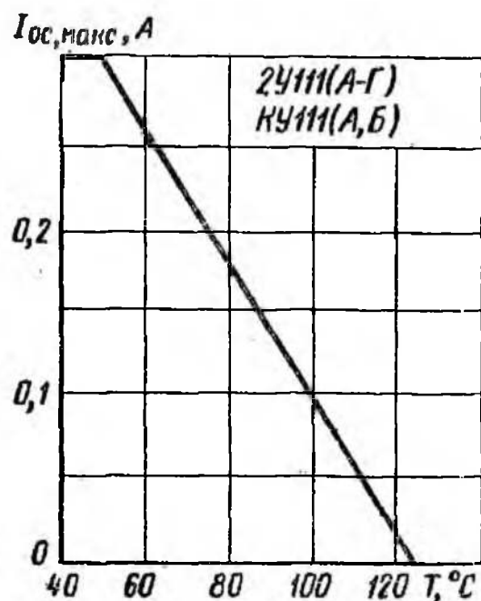
Зависимость допустимого постоянного тока в открытом состоянии от температуры
