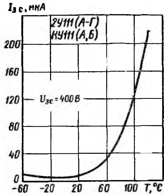
Зависимость тока в закрытом состоянии от температуры
