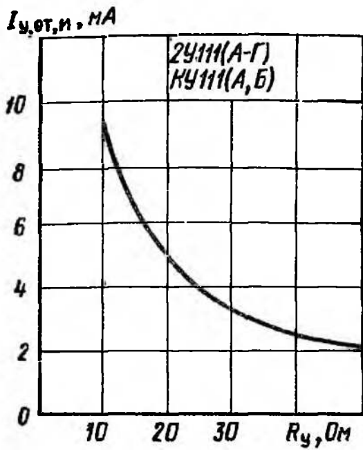
Зависимость отпирающего импульсного тока от сопротивления резистора в цепи управления.
