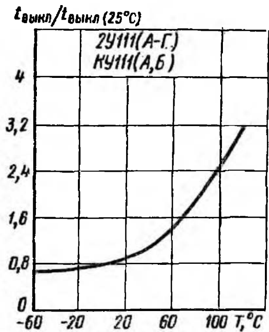
Зависимость времени выключения от температуры
