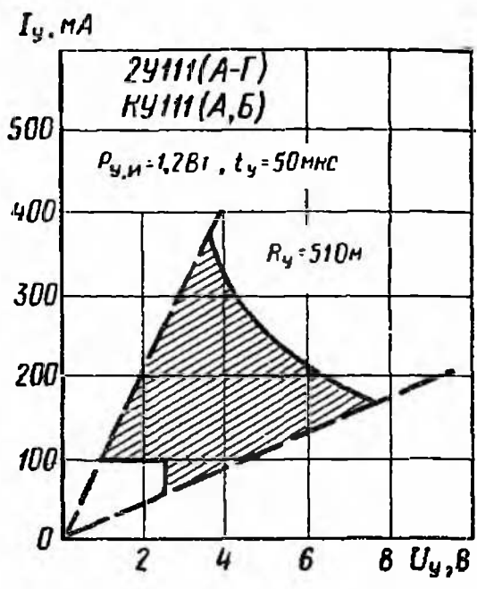
Диаграмма управления. Заштрихована область разрешенных значений
