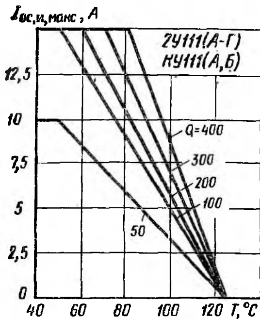
Зависимости допустимого импульсного тока в открытом состоянии от температуры
