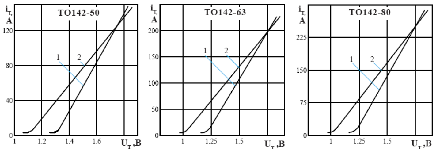
Рисунок 1 - Предельная вольтамперная характеристика в открытом состоянии при температуре перехода 25 °С (1) и максимальной температуре перехода T_{jm} (2) I_T = 3,14I_{TAVM}
