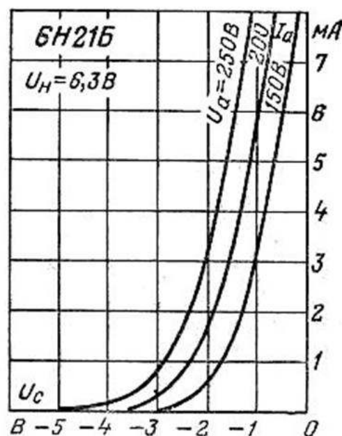
Анодно-сеточные характеристики.
