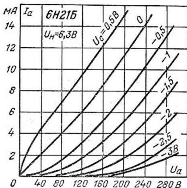
Анодные характеристики.
