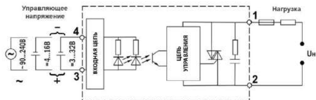
СХЕМА ПОДКЛЮЧЕНИЯ
