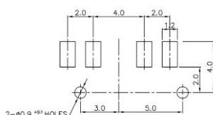
Схема установки
